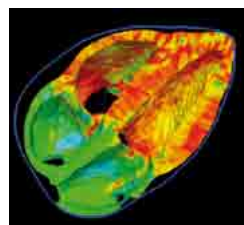
Darstellungen im Rahmen der Entwicklung eines Modells für das elektrome- chanische System im Herzen Representations for the development of a model of the electromechanical system of the heart
